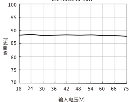
效率Vs输入电压(满载) URA4815MD-10W
