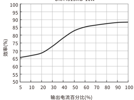
效率Vs输出负载(Vin=48V) URA4815MD-10W
