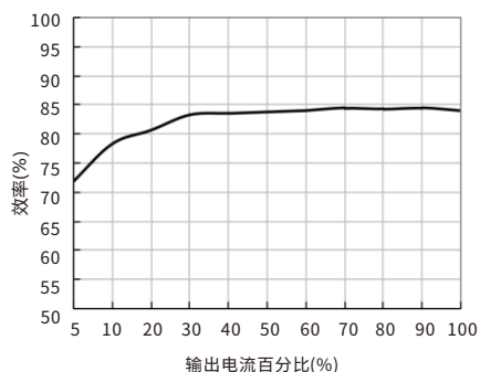
效率Vs输出负载(Vin=24V) URB2405MD-10W
