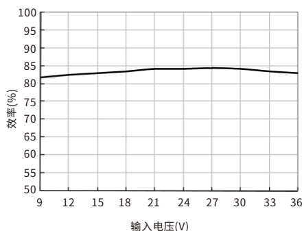
效率Vs输入电压(满载) URF2405MD-10W
